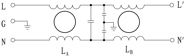
原理图
