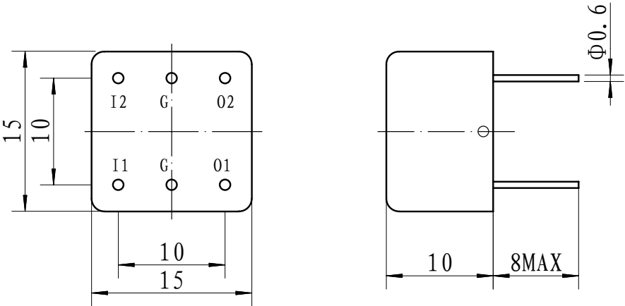
外形尺寸图
