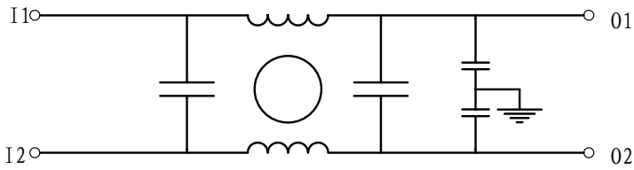
原理图
