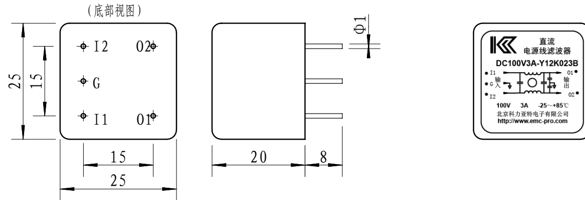
外形尺寸图
