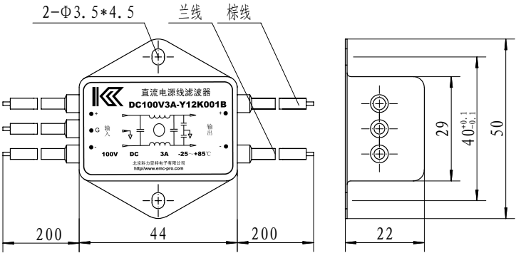
外形尺寸图
