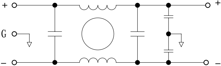
原理图
