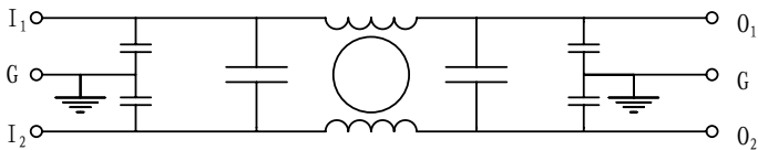
原理图
