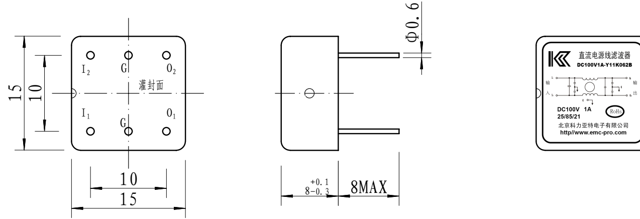
外形尺寸图
