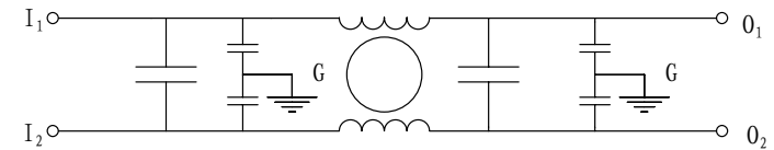
原理图
