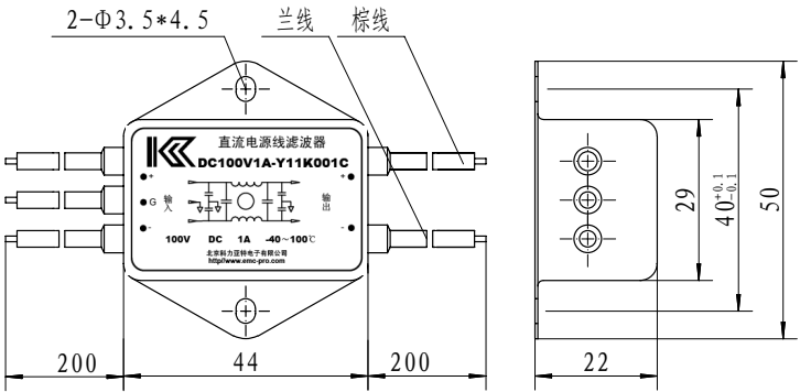
外形尺寸图
