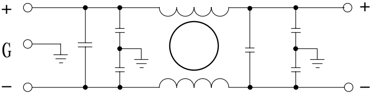
原理图
