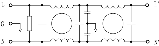
原理图
