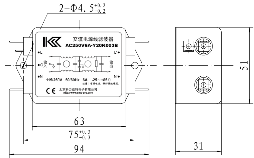
外形尺寸图
