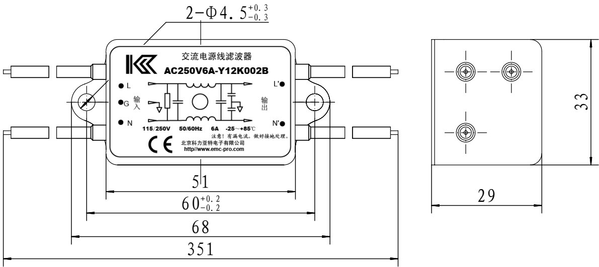
外形尺寸图
