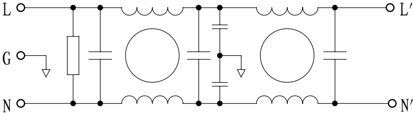
原理图
