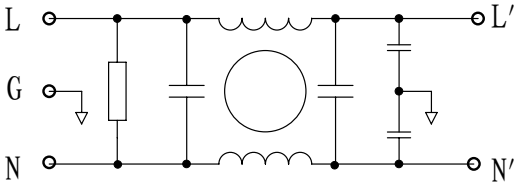
原理图
