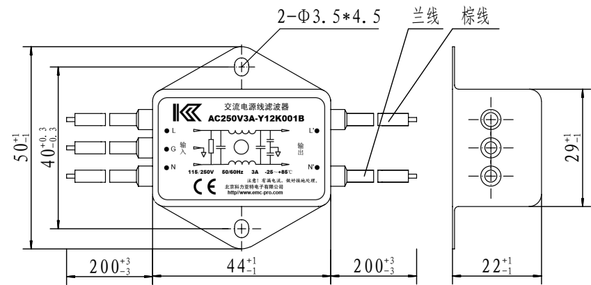
外形尺寸图
