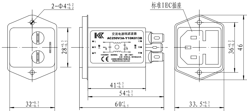
外形尺寸图
