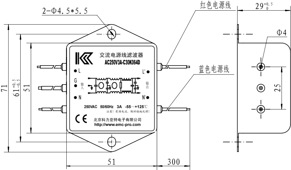
外形尺寸图
