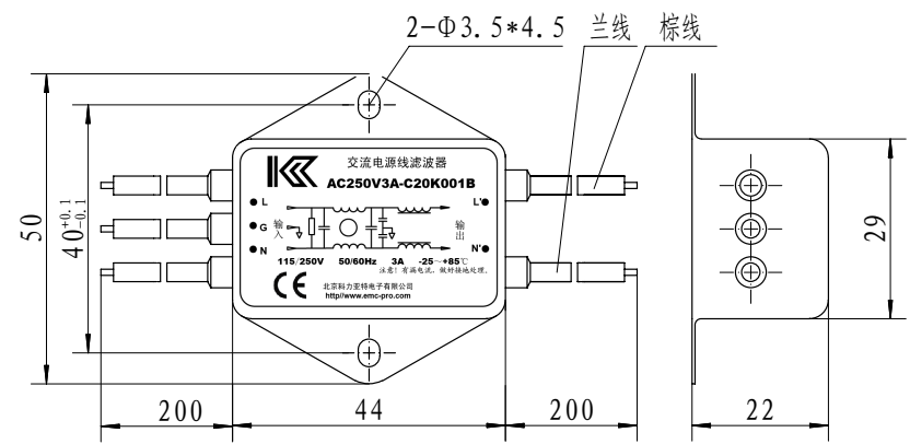
外形尺寸图
