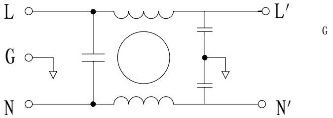
原理图
