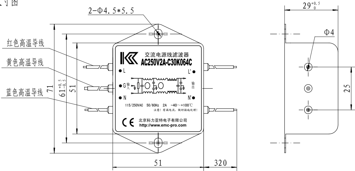
外形尺寸图
