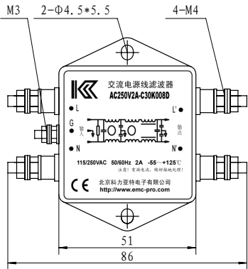
外形尺寸图
