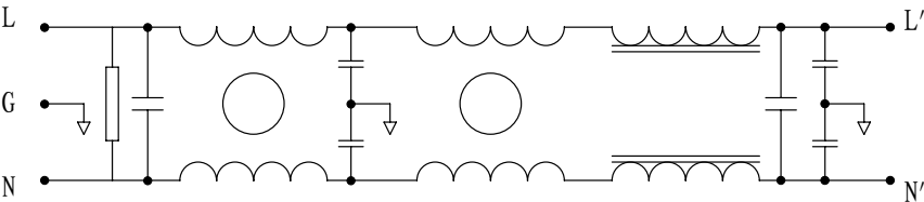
原理图
