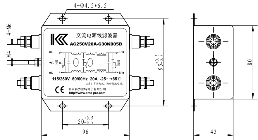
外形尺寸图
