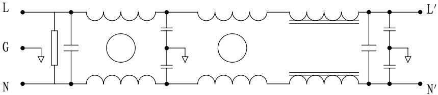
原理图
