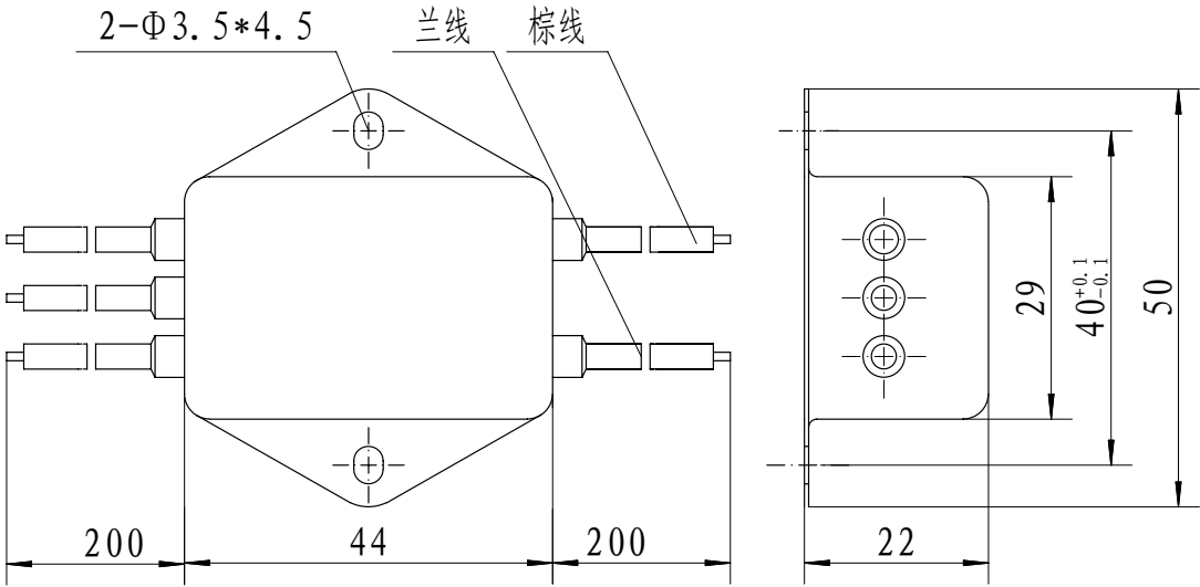
外形尺寸图
