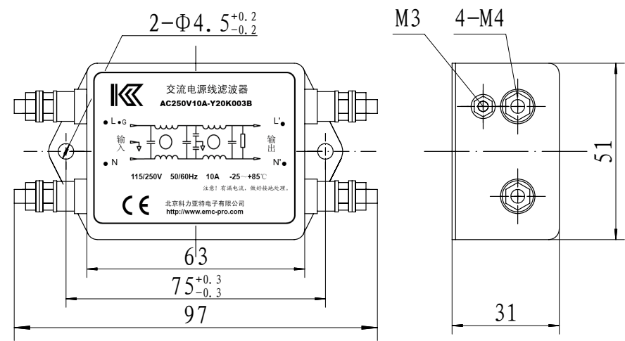
外形尺寸图
