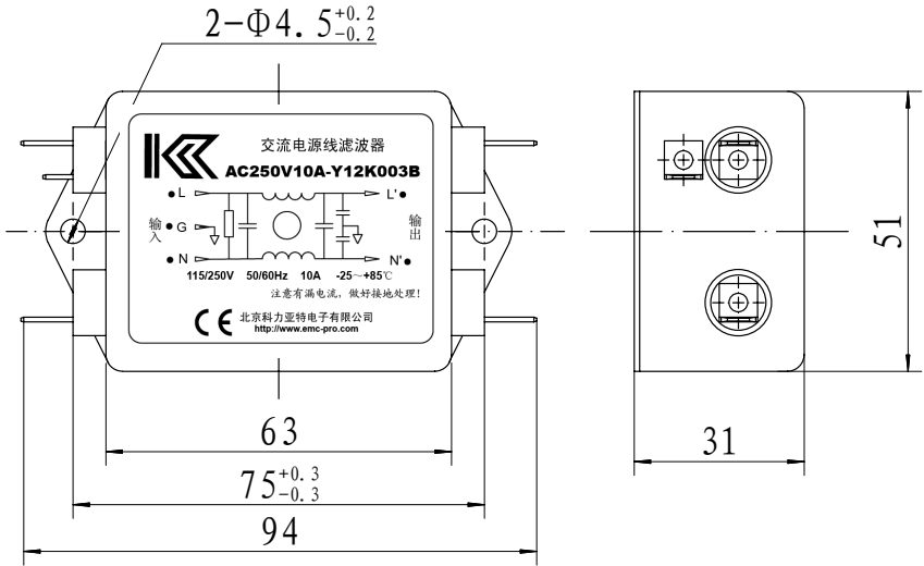
外形尺寸图
