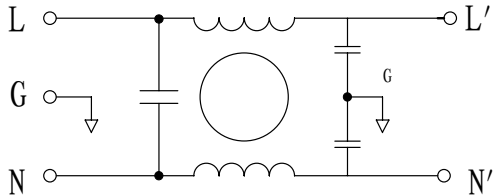
原理图
