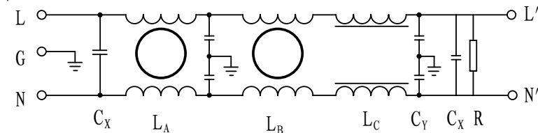
原理图
