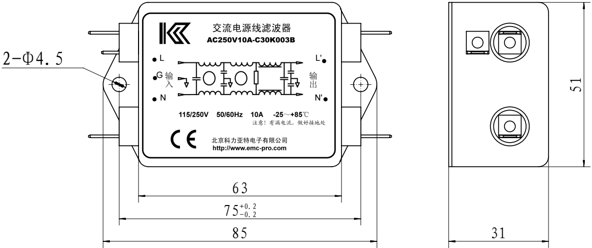
外形尺寸图
