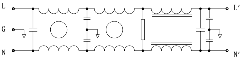
原理图
